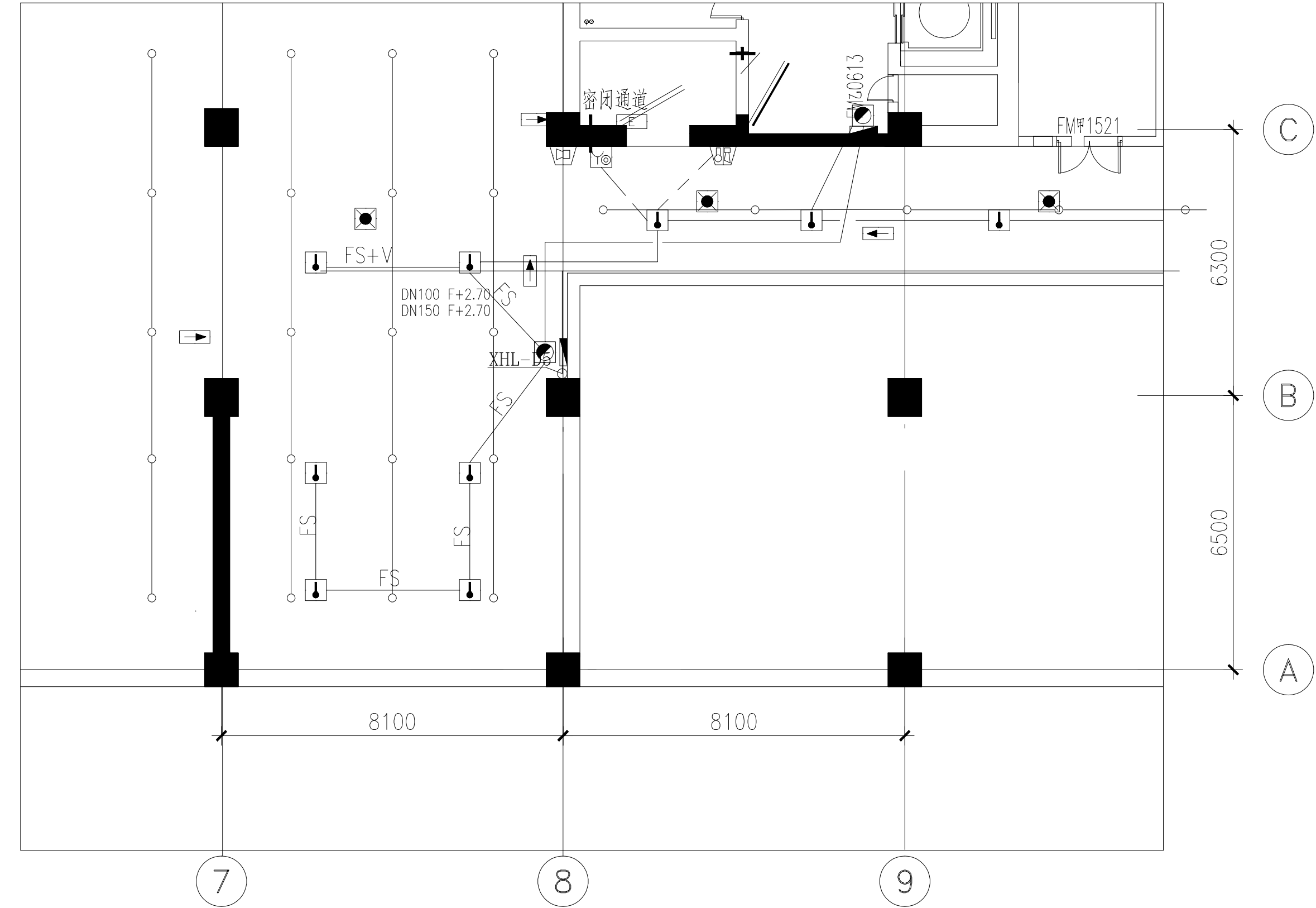
原始消防布置图 SCALE 1:100
