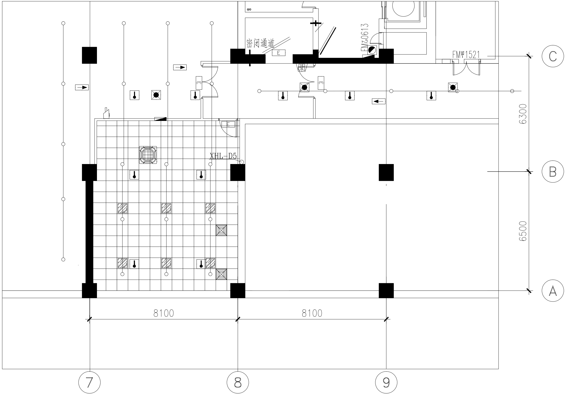
消防改造布置图 SCALE 1:100
