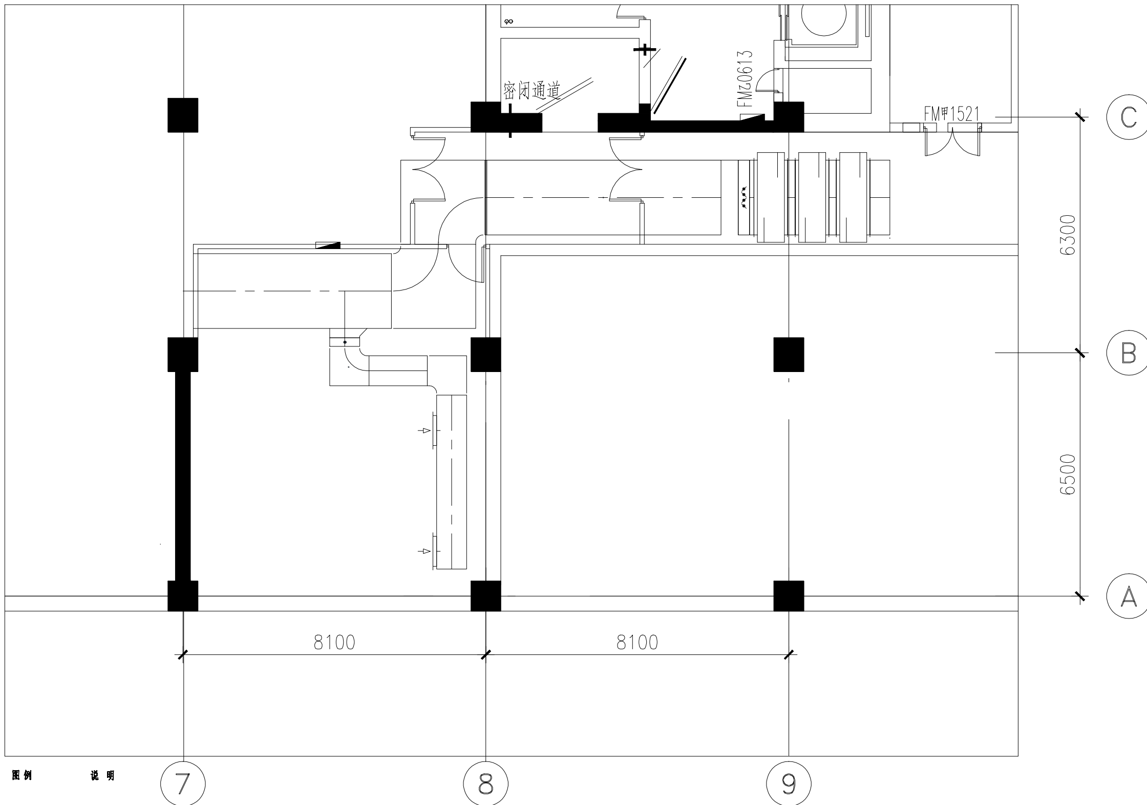
PLANE 骨科手术机器人测试区排风平面图 SCALE:1:50
